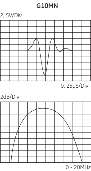
リアルタイム波形と周波数スペクトラム
